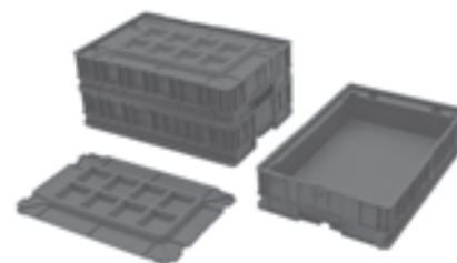
P 2006 (C KLT-6414) Tampa opcional Fundo lego e parede dupla
